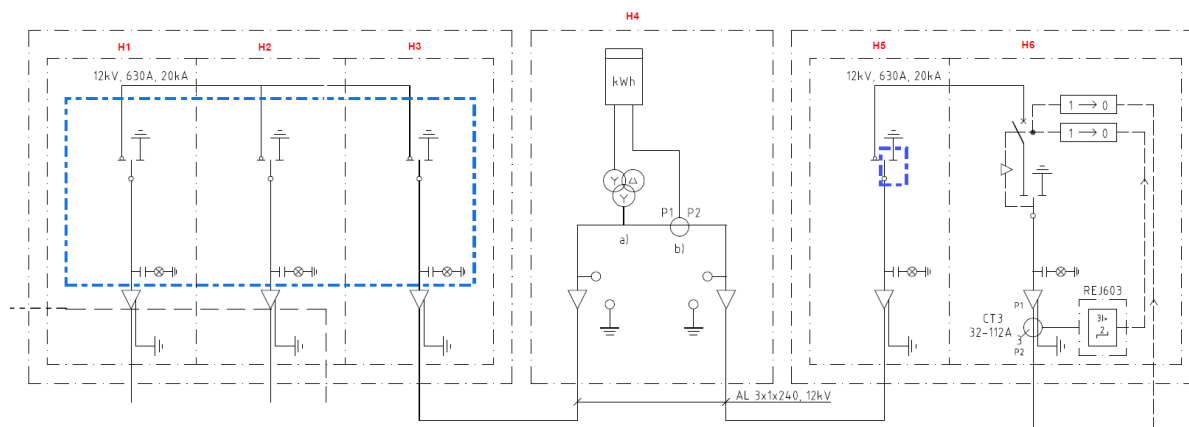
Bild 1. Principskiss för enlinjeschema
