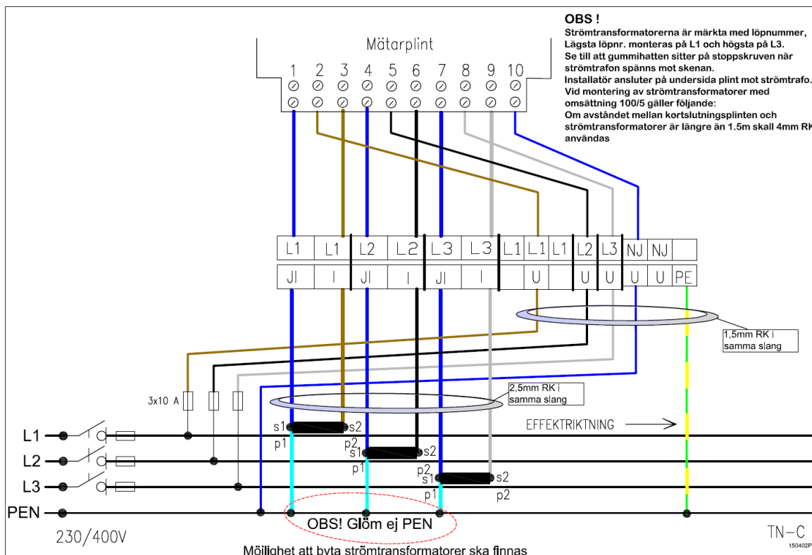
Figur 18 Exempel på förbindningsschema för mätutrustning med strömtransformator, TN-C
