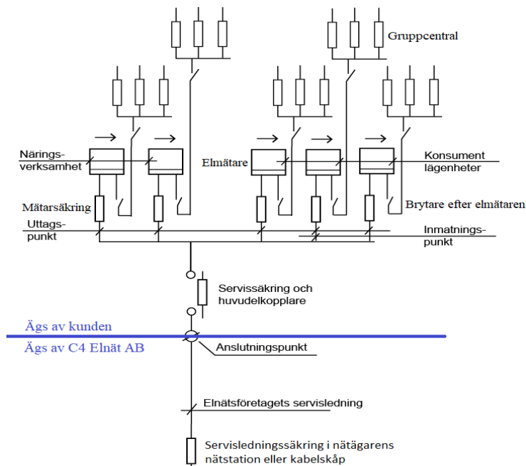
Figur 3 Exempel på flera mätarplatser
