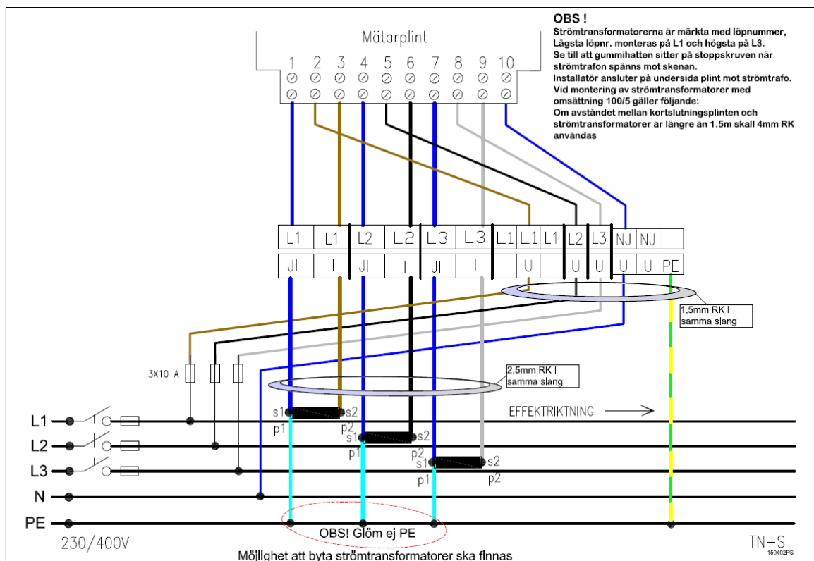
Figur 19 Exempel på förbindningsschema för mätutrustning med strömtransformator, TN-S
