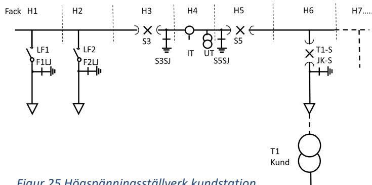
Figur 25 Högsämningsställverk kundstation
