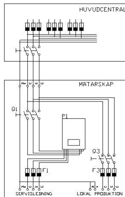
Figur 22 Ex med nytt mätarskåp
