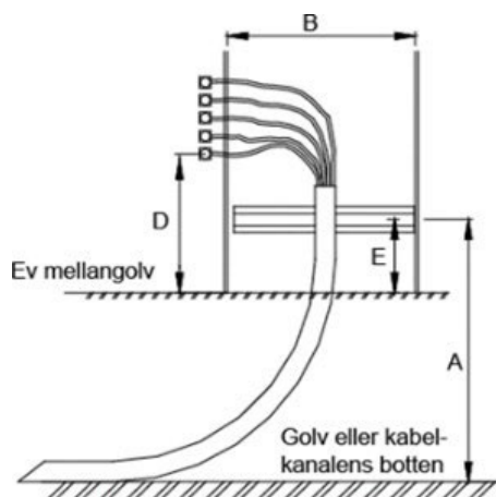
Figur 6 – Utrymme för servisledning vid skåpkopplingsutrustning
