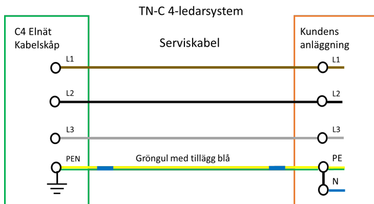
Figur 8 Elanslutning TN-C
