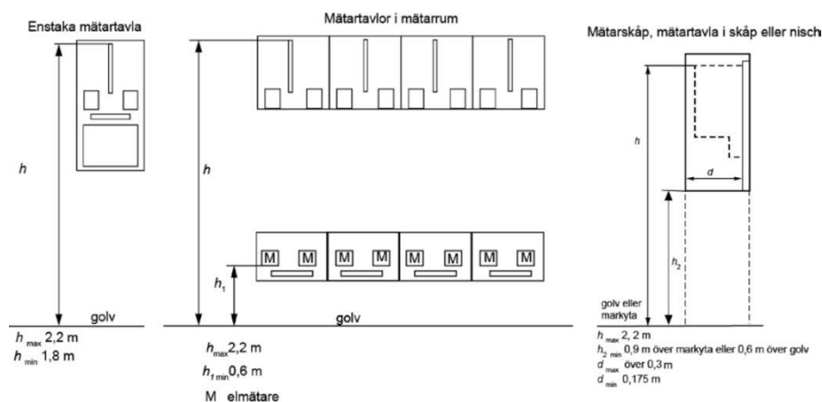
Figur 12 Mätartavlor
