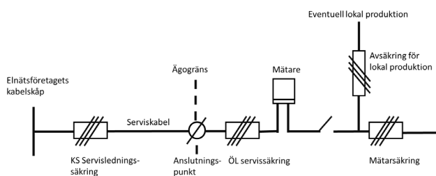
Figur 20 Exempel produktionsanläggning
