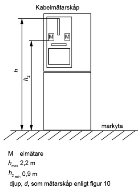
Figur 14-Markmätarskåp 80A - 1500A med mätartavla enligt SS 430 01 15
