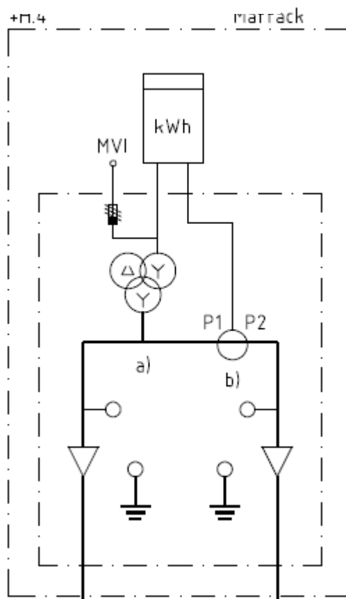
Figur 26 Trefasgrupp i H4 mätacket.
