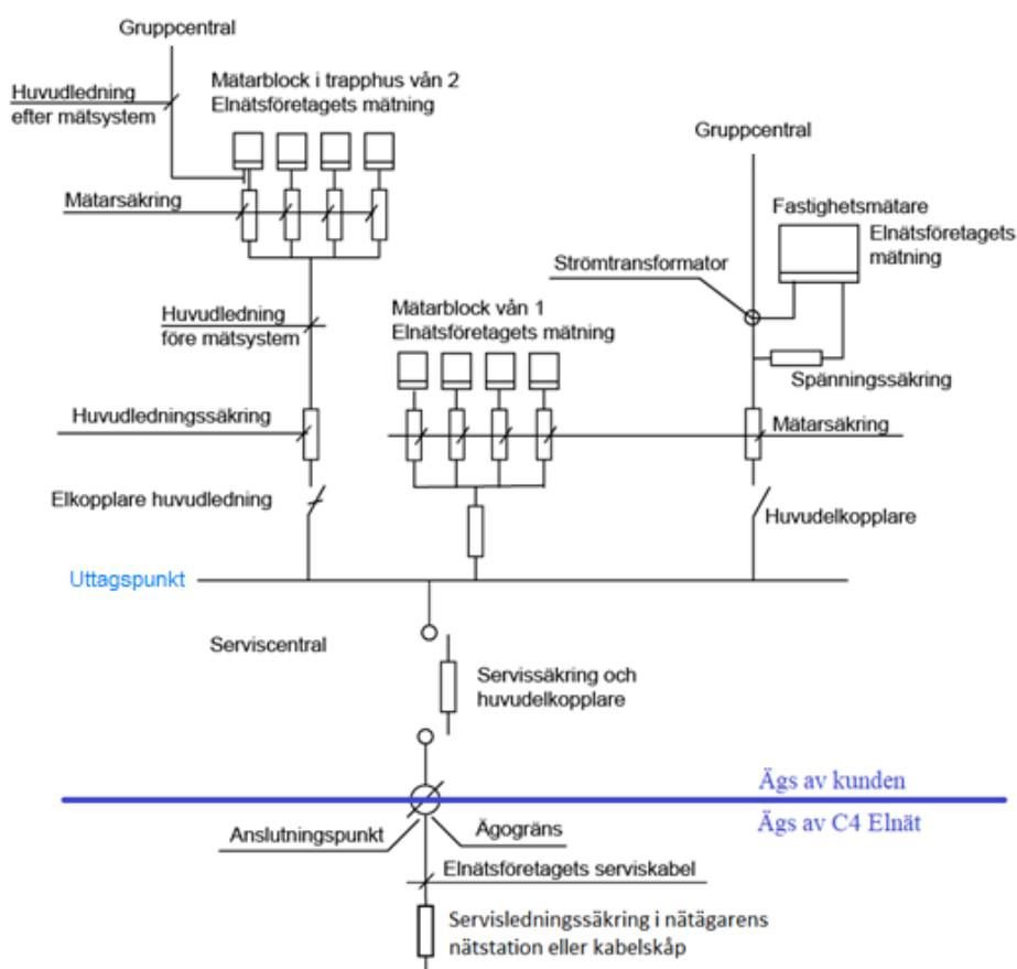
Exempel på benämningar i elinstallationen
