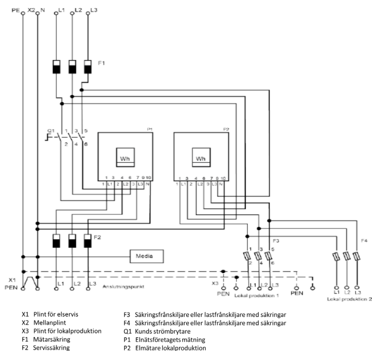
Figur 21 TN-C-S anläggning med produktion större än mätarsäkring 16 A – 63 A, samt med inmatning med två enheter för lokal produktion
