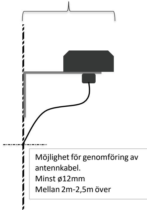
Figur 27 Fäste till antenn för mätsignal.
